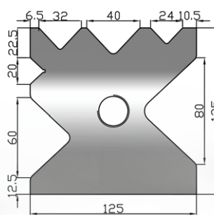
USH M125 V20-24-32-40-60-80/86°
