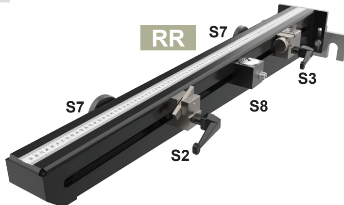
Riferimento in lamiera. Si consiglia l'applicazione su presse piegatrici tipo AMADA/SCHIAVI (L.mm 500-1000-1500) Sheet reference. The use is recommended on AMADA / SCHIAVI press brakes type (L.mm 500-1000-1500)
