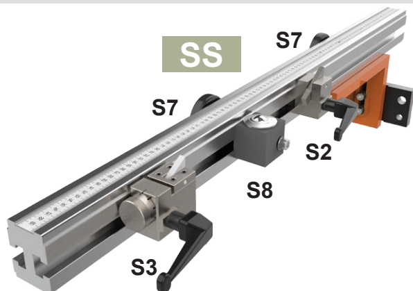
Riferimento in acciaio regolabile in altezza. E' applicabile a qualsiasi tipo di pressa piegatrice Steel reference. The height is adjustable and it can be used on any type of press brake
