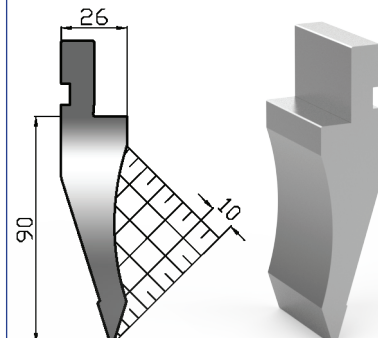
US 112/35° R0,8 h 90 mm
