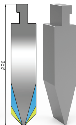
USH 220 B 86°60°30° R2,0
