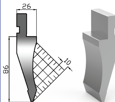
US 112/35° R1,5 h 86 mm
