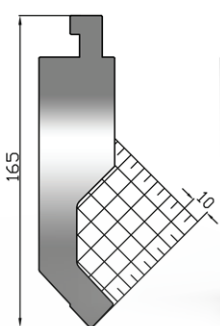
USH 165 A 86° R1,5
