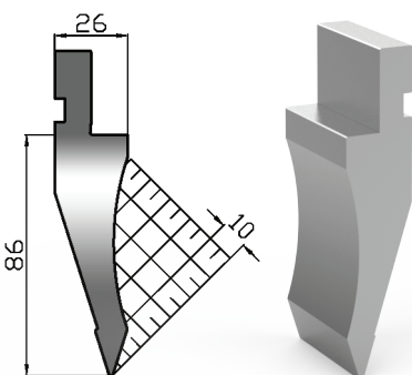
US 112/35° R0,8 h 86 mm
