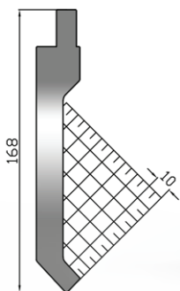
USH 168 A 86° R1,5
